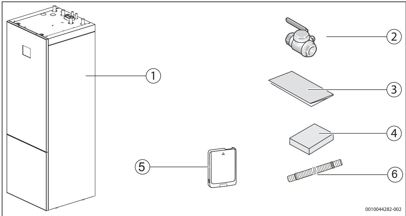
Bild 1 Lieferumfang
