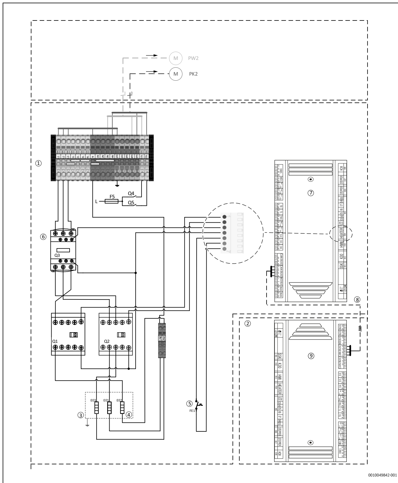
Bild 59 Spannungsversorgung Inneneinheit
