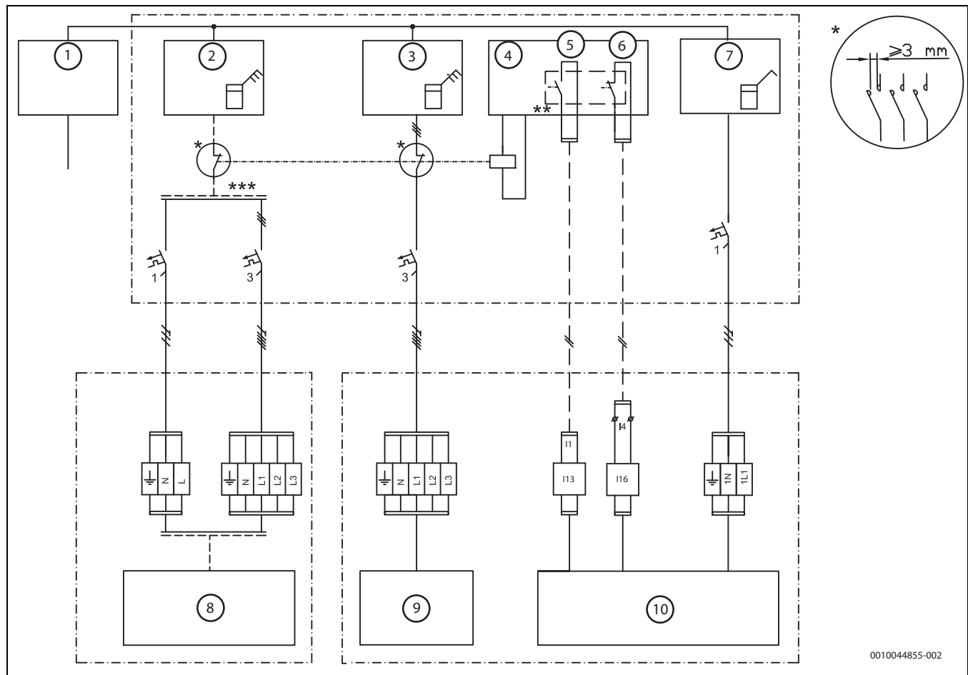
Bild 49 Alternative Lösung
