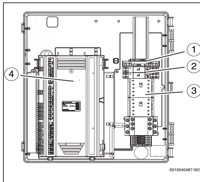
Bild 40 Anordnung der Komponenten im Klemmenkasten
