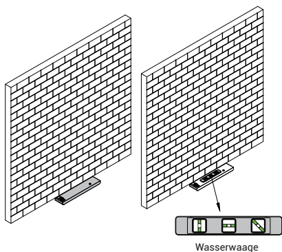
Wasserwaage
