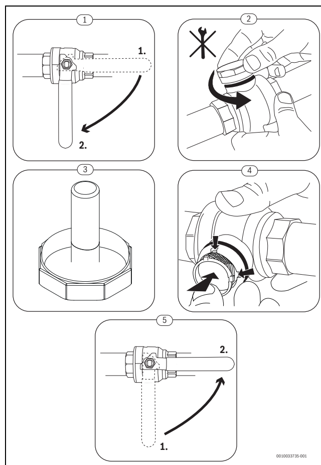
Bild 12 Siebreinigung
