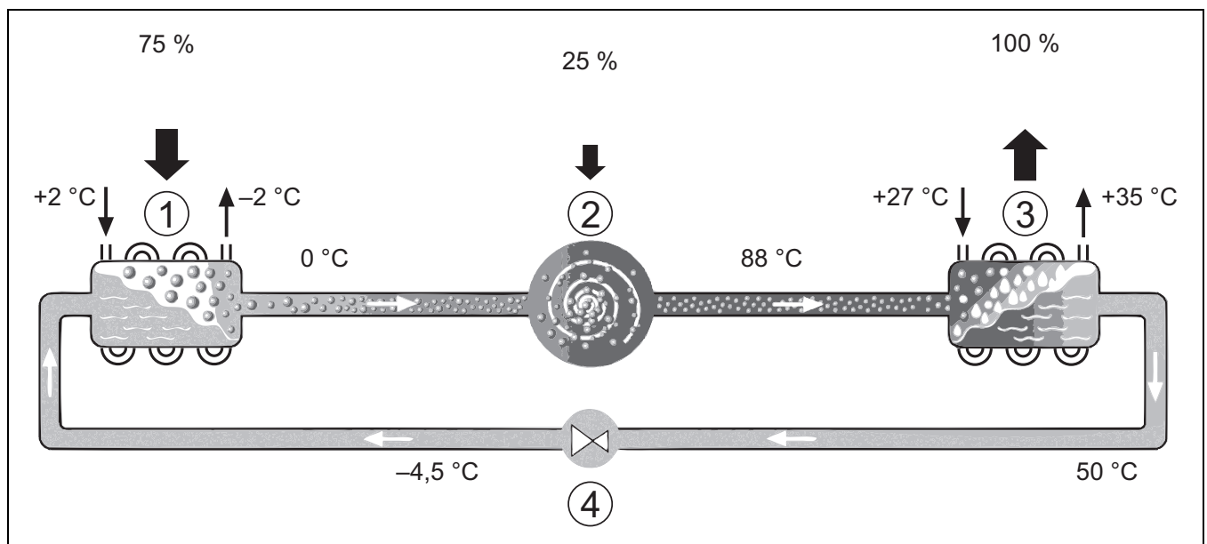
Bild 4 Funktionsprinzip des Kältemittelkreises in der Wärmepumpe
