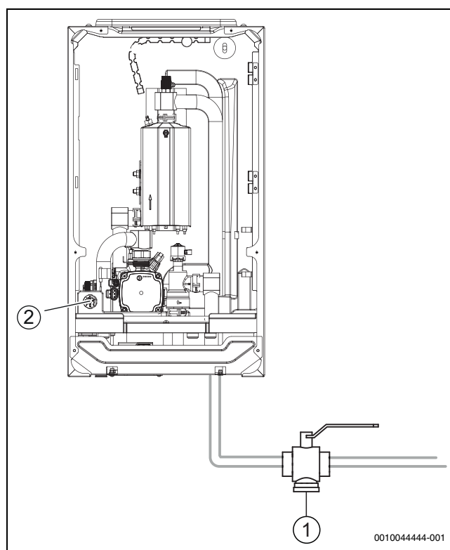
Bild 11 Inneneinheit Logatherm WLW176i/186i E
