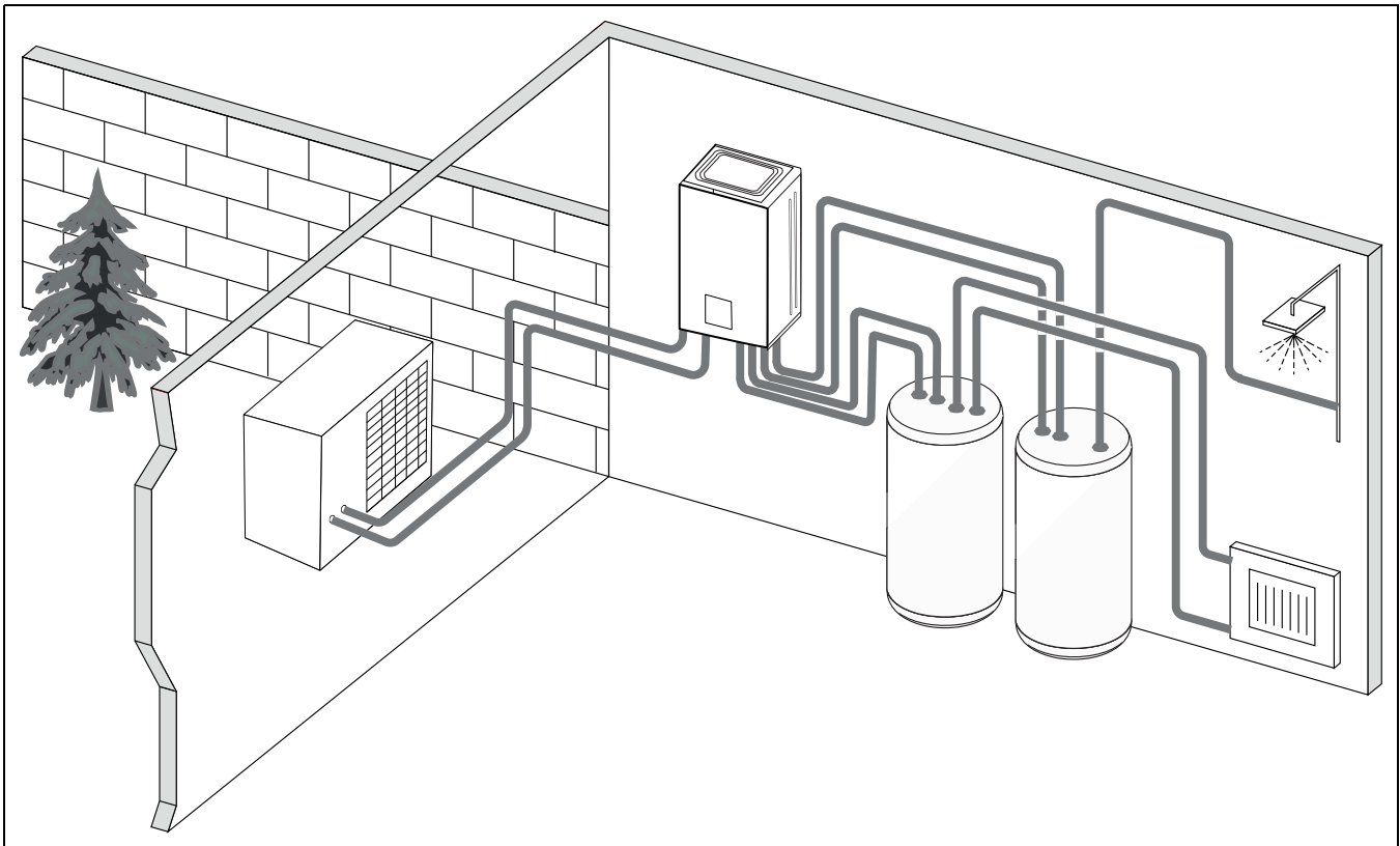
Bild 5 Wärmepumpe Logatherm WLW MB AR, Inneneinheit Logatherm WLW176i/186i E mit elektrischem Zuheizter und externem Warmwasserspeicher
