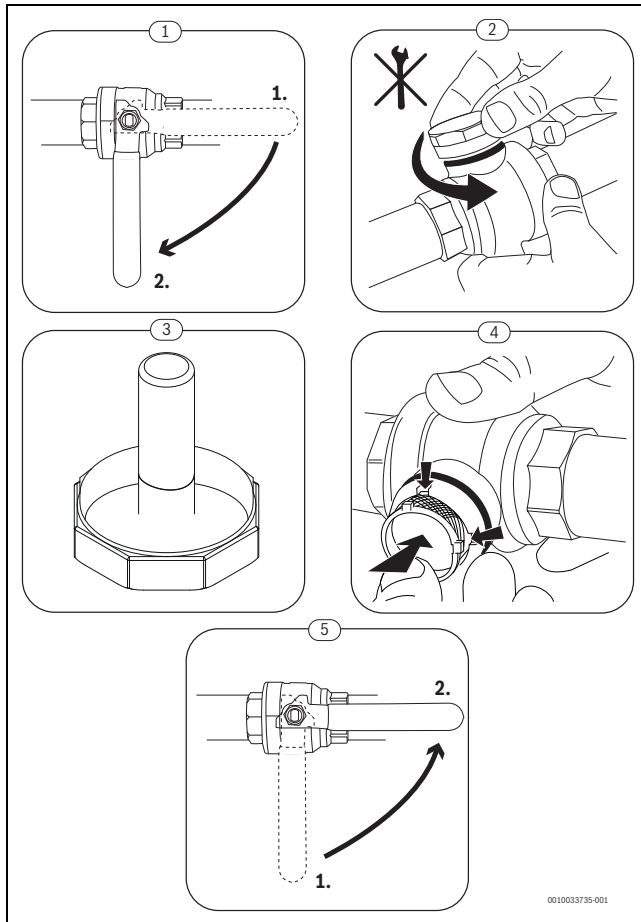
Bild 46 Siebreinigung
