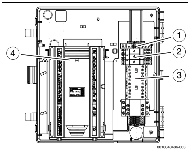
Bild 34 Anordnung der Bauteile im Klemmenkasten
