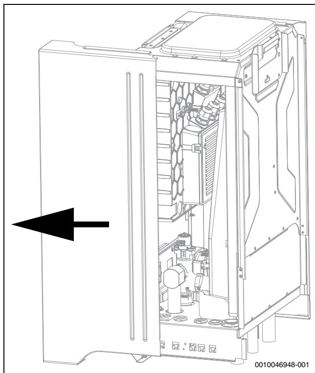
Bild 18 Seitliche Abdeckung entfernen
