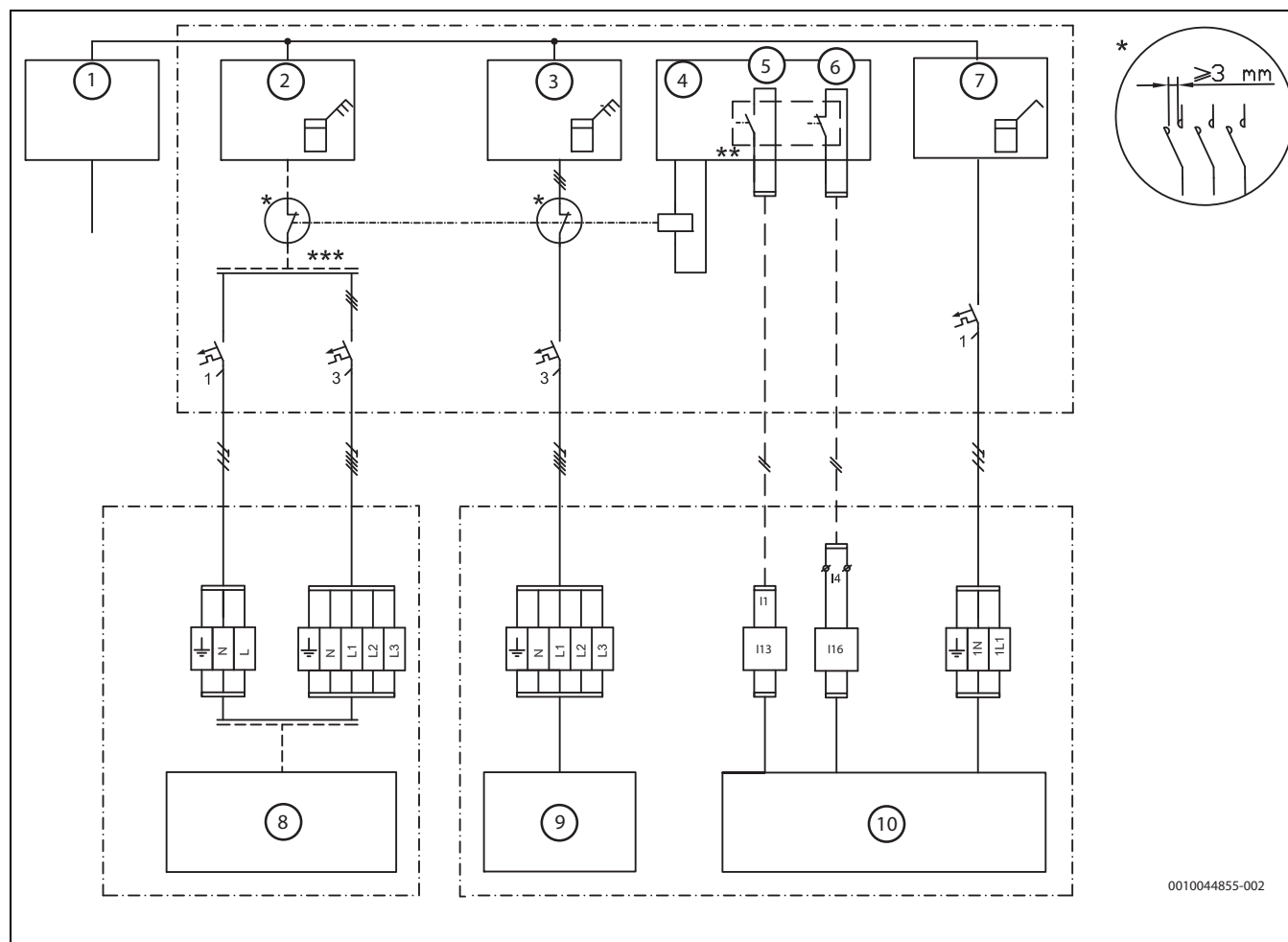
Bild 44 Alternative Lösung
