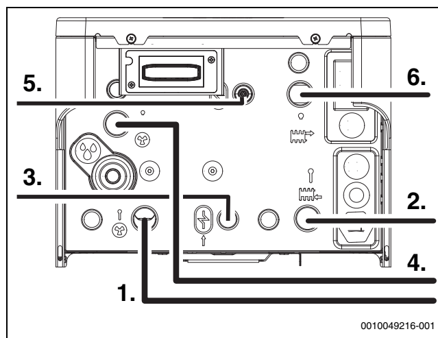
Bild 19 Rohranschlüsse
