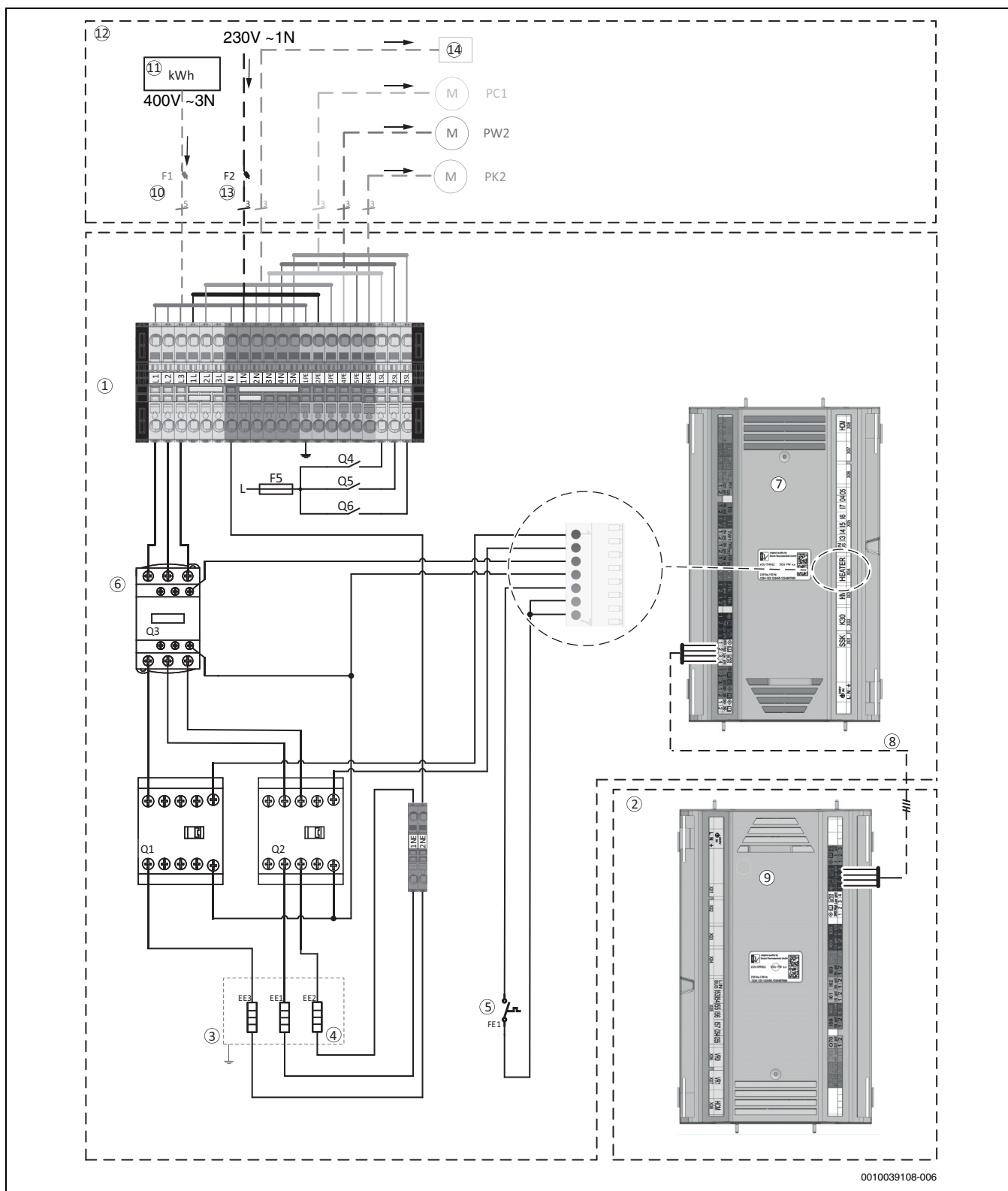
Bild 53 Spannungsversorgung Inneneinheit, EVU-Sperre
