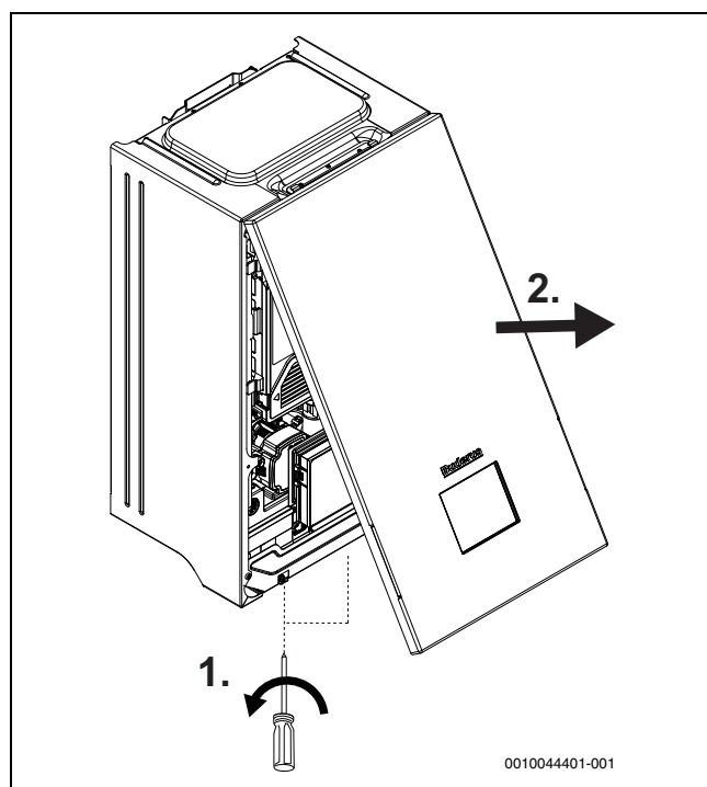
Bild 15 Frontplatten abnehmen
