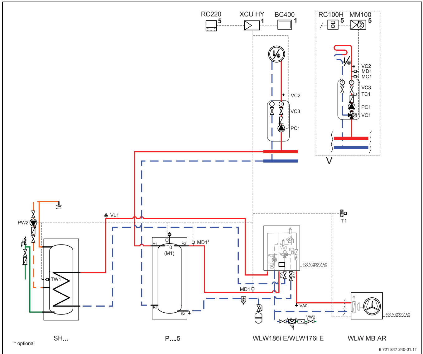
Bild 48 Wärmepumpe, Inneneinheit, Pufferspeicher und Warmwasserbereiter
