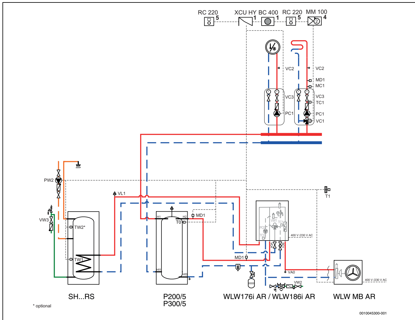
Bild 49 Wärmepumpe, zwei Heizkreise, Inneneinheit, Pufferspeicher und Warmwasserspeicher
