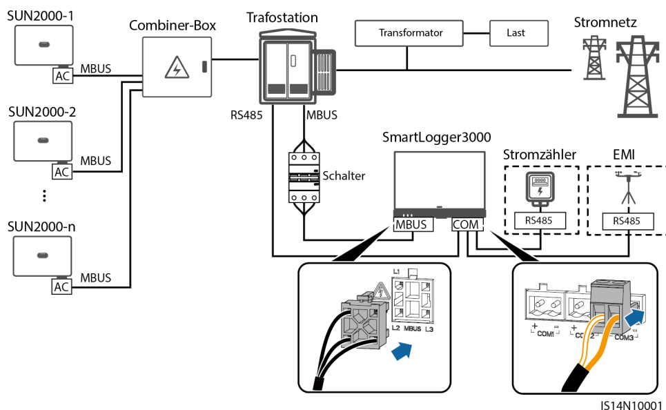
Abbildung 5-24 MBUS-Kommunikation (Großanlagen-Szenario)
