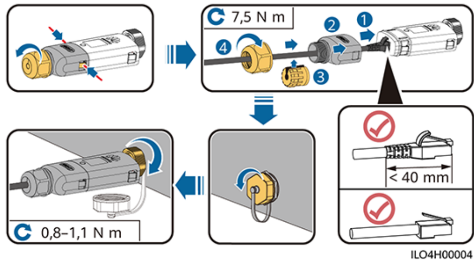
Abbildung 5-19 Anschließen des WLAN-FE Smart Dongle (FE-Kommunikation)
