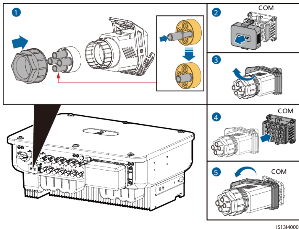
Abbildung 5-21 Anschließen des Signalkabelsteckers
