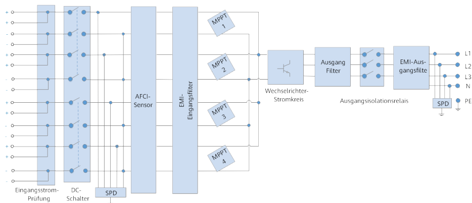
Abbildung 2-5 Schematisches Diagramm
