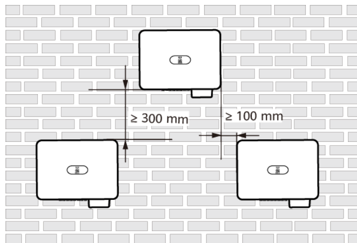
Abbildung 4-4 Zweischichtiger Dreiecksmontagemodus (empfohlen)
