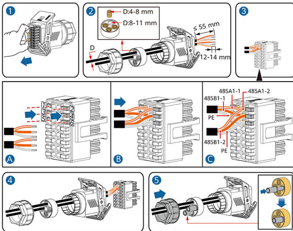
Abbildung 5-26 Anschließen des Kabels
