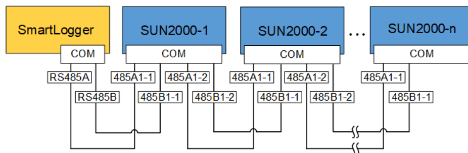
Abbildung 5-23 SmartLogger-Netzwerkaufbau
