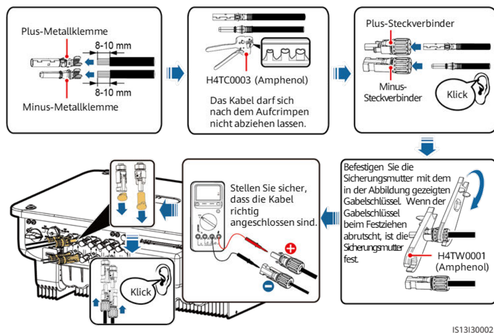
Abbildung 5-13 Anschließen der DC-Stromkabel
