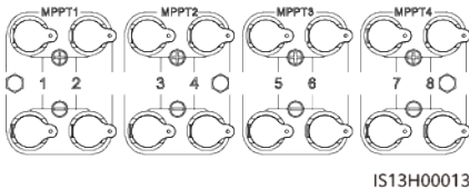
Abbildung 5-12 DC-Eingangsklemmen
