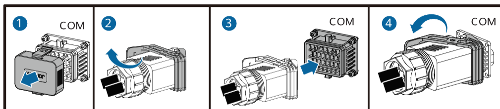
Abbildung 5-27 Sichern des Signalkabelsteckers
