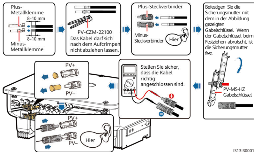
Abbildung 5-15 Anschließen der DC-Stromkabel
