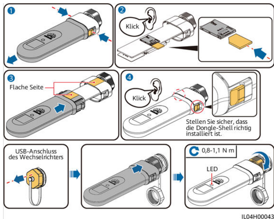
Abbildung 5-17 Installation des 4G Smart Dongle (SDongleB-06)
