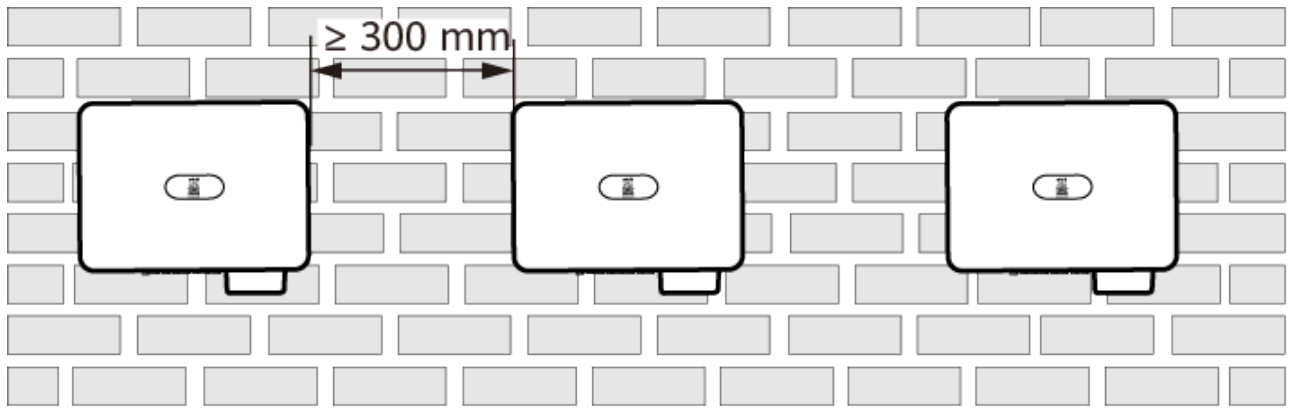
Abbildung 4-3 Horizontaler Montagemodus (empfohlen)
