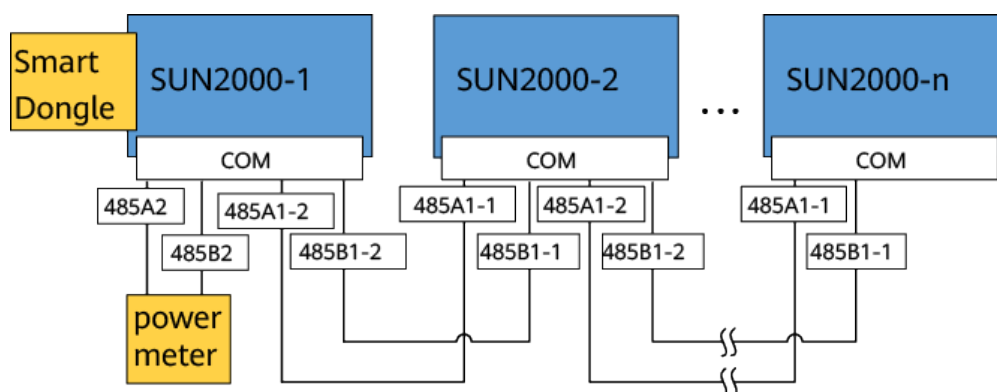
Abbildung 5-22 Smart Dongle-Netzwerkaufbau
