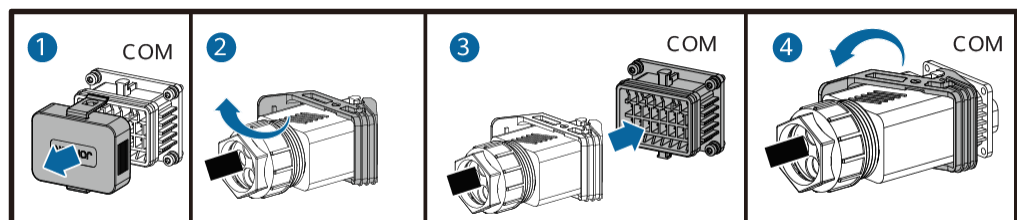
Abbildung 5-29 Sichern des Signalkabelsteckers
