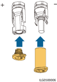
Abbildung 5-14 Verschlussstopfen
