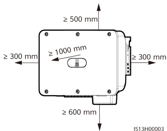
Abbildung 4-2 Abstände
