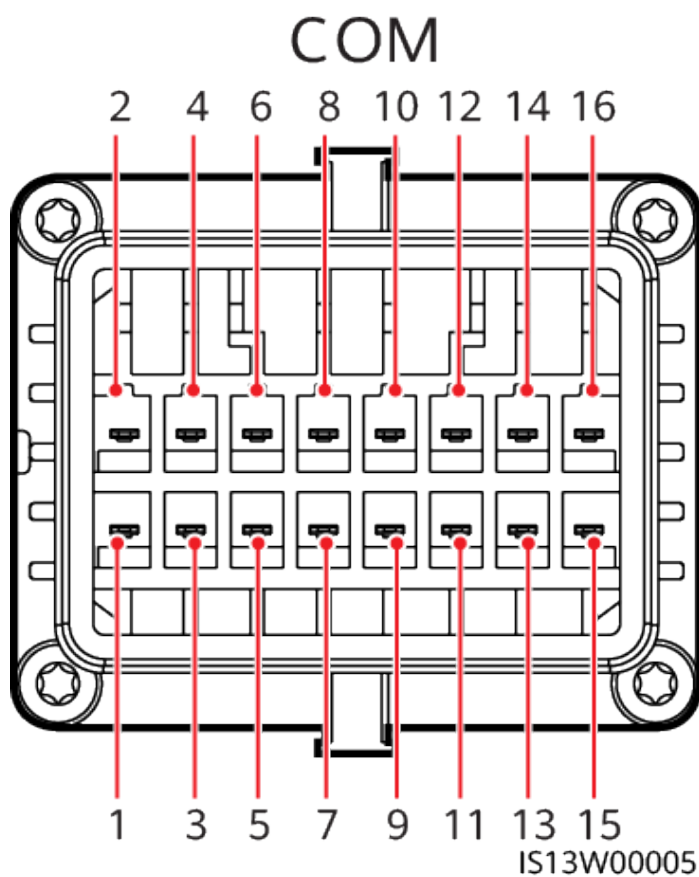
Abbildung 5-20 Pin-Definitionen
