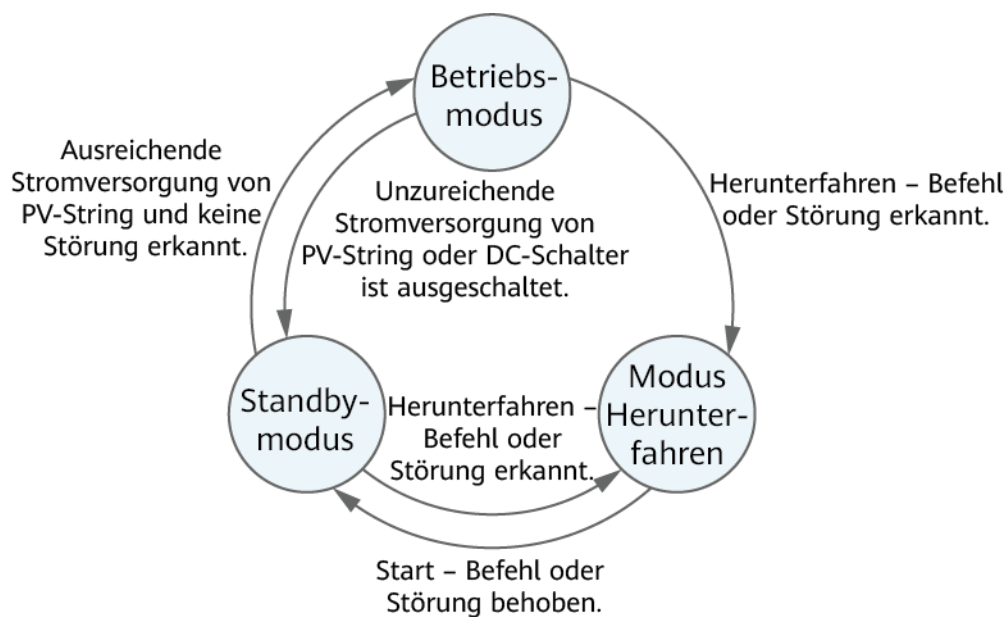
Abbildung 2-6 Arbeitsmodi
