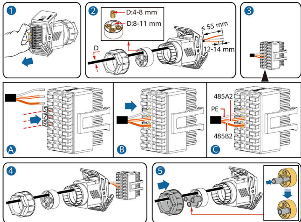
Abbildung 5-28 Installieren des Kabels
